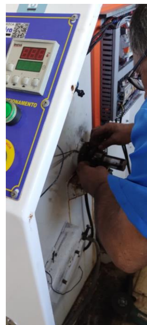
Fotos 14 a 19: Sequência fotográfica evidenciando a retirada do maquinário da lavanderia industrial para reparo no Lar dos Idosos (Erval Velho).
