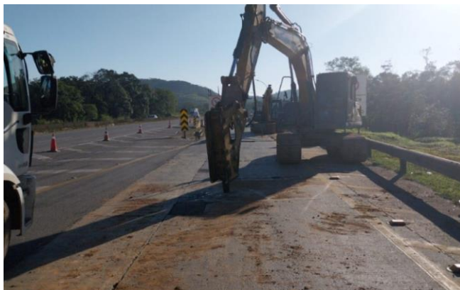
Figura 01 – Recuperação do pavimento – Balança Garuva/SC
