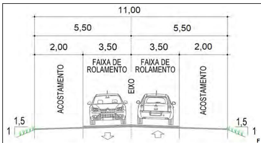
Figura 1 – Seção tipo projetada para o Lote A
