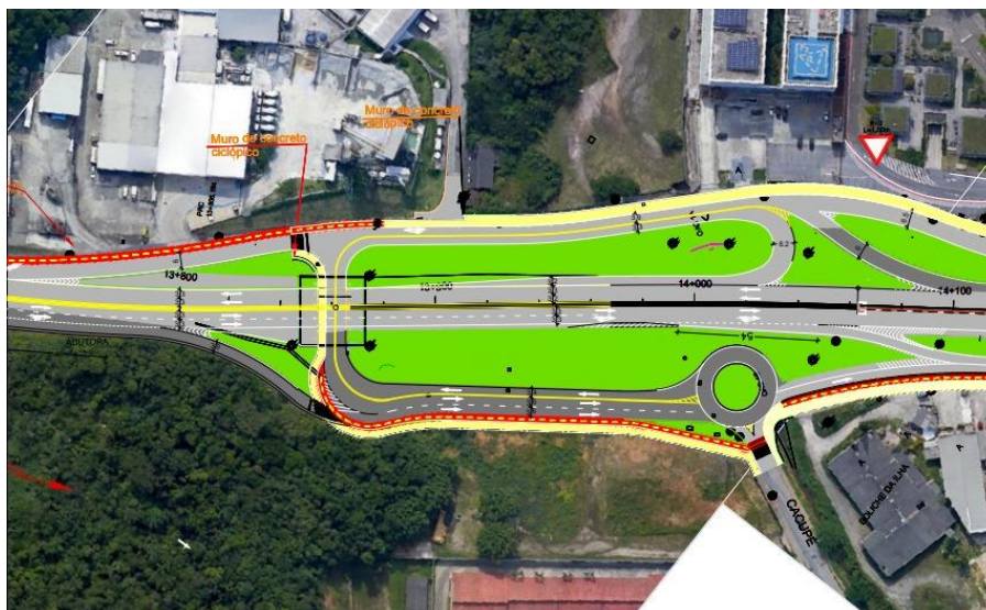
Figura 5 – Melhorias no acesso de Cacupé
