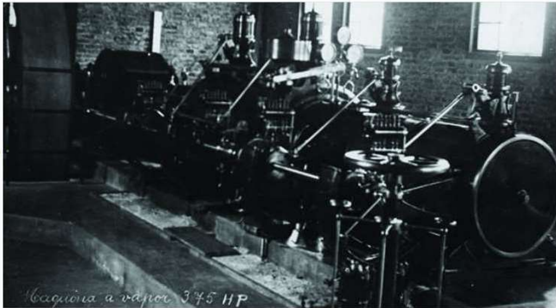
1943: Vargem Bonita - Primeira máquina a vapor
