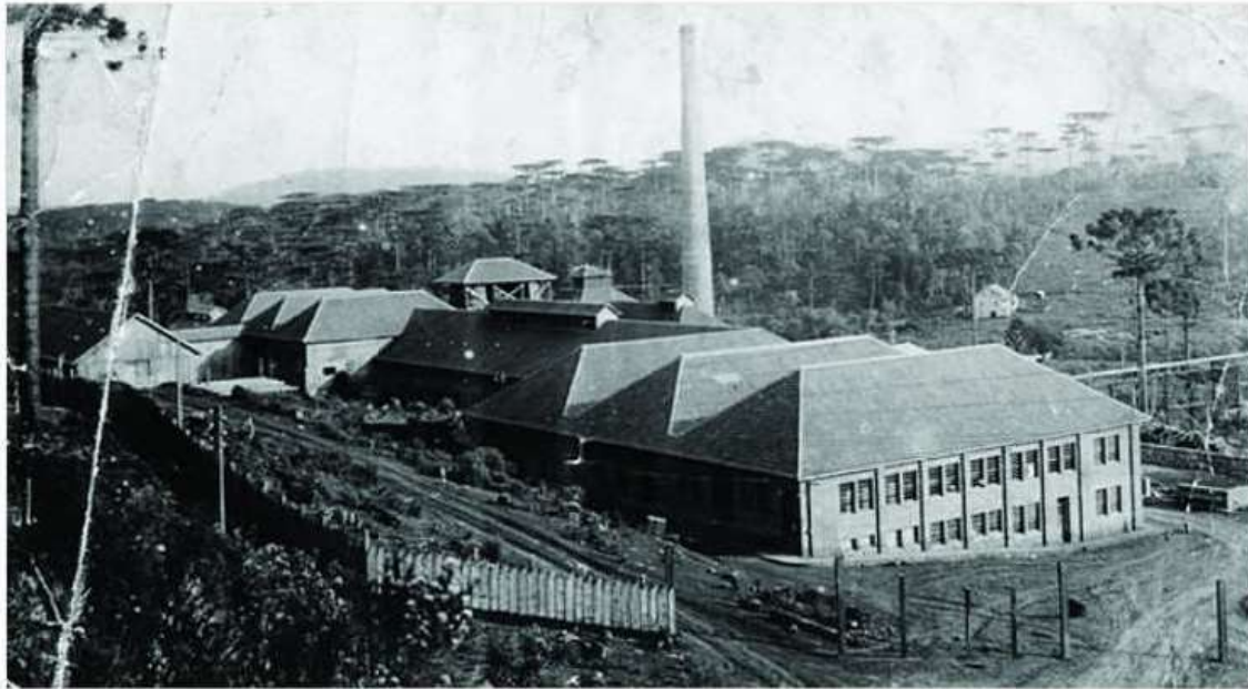
1944: Vargem Bonita - Vista geral da fábrica
