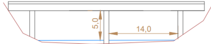
Figura 1 - Croqui longitudinal da ponte.
